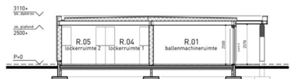
Doorsnede B
