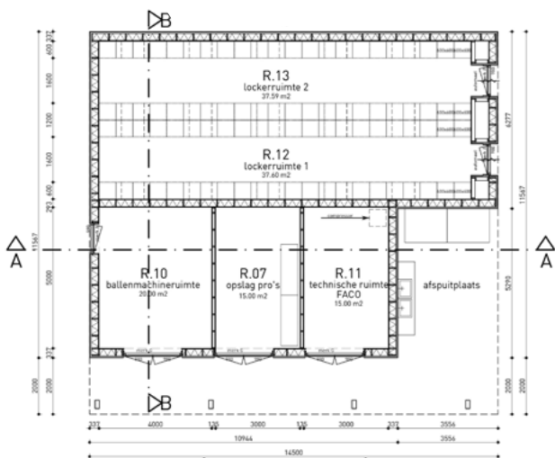
Begane grond
