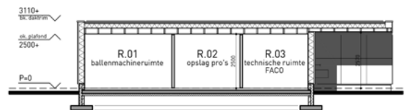
Doorsnede A
